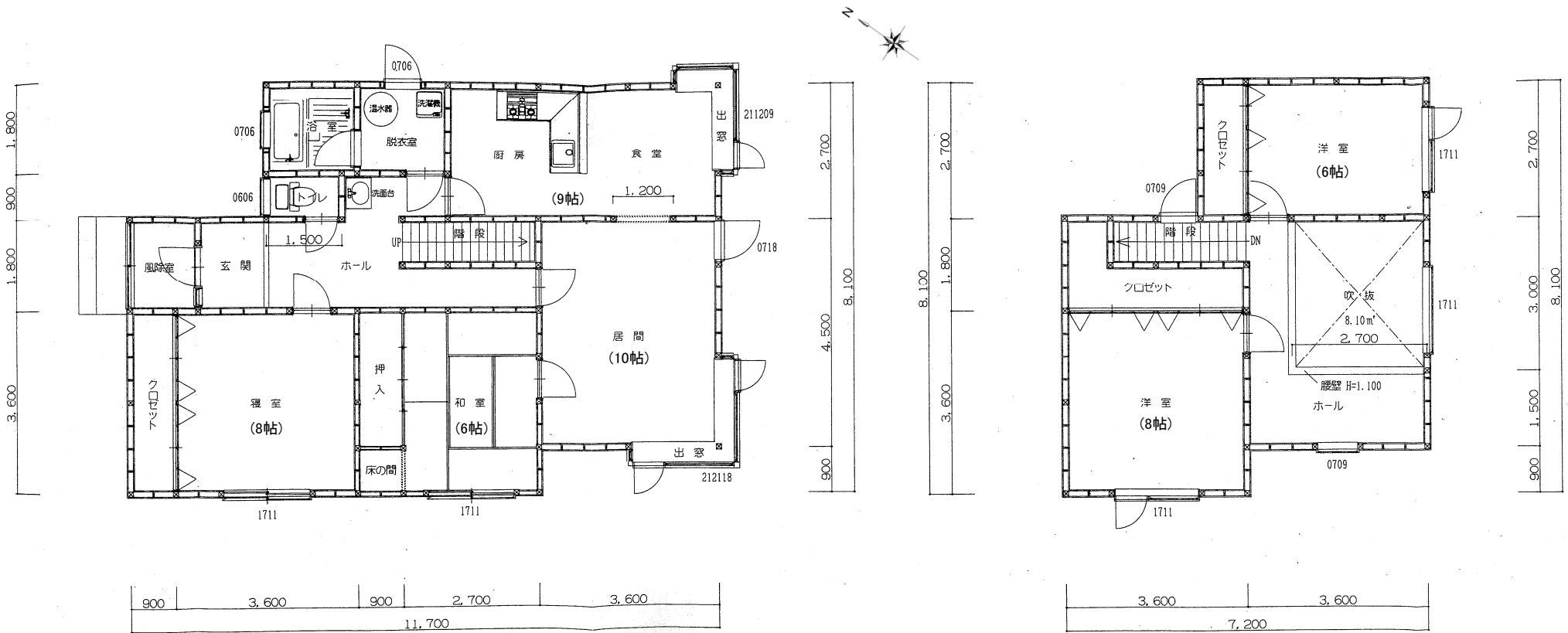
1階平面図
