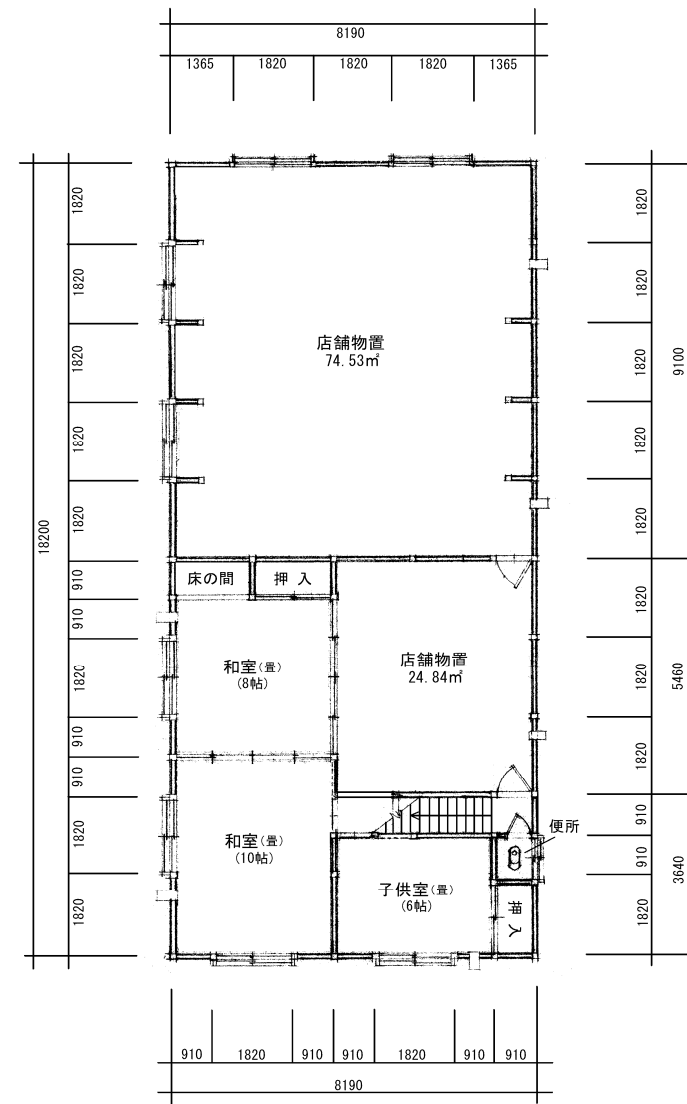
《 2階平面図 》
