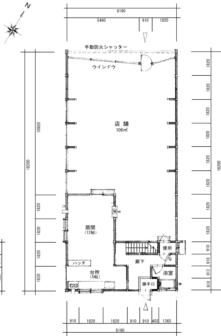
《 1階平面図 》
